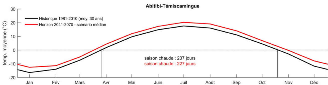
Figure 3 : évolution de la température moyenne mensuelle, en climat historique et futur. La saison dite « chaude », avec une température moyenne supérieure à 0 °C, serait allongée de 20 jours dans le scénario médian.
