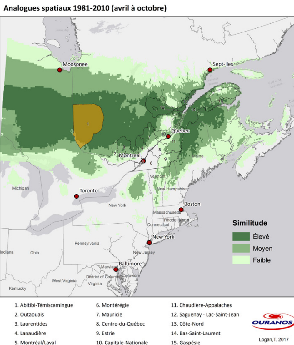
Figure 5 : analogues spatiaux du climat de l’Abitibi-Témiscamingue établi pour la période 1981-2010.
