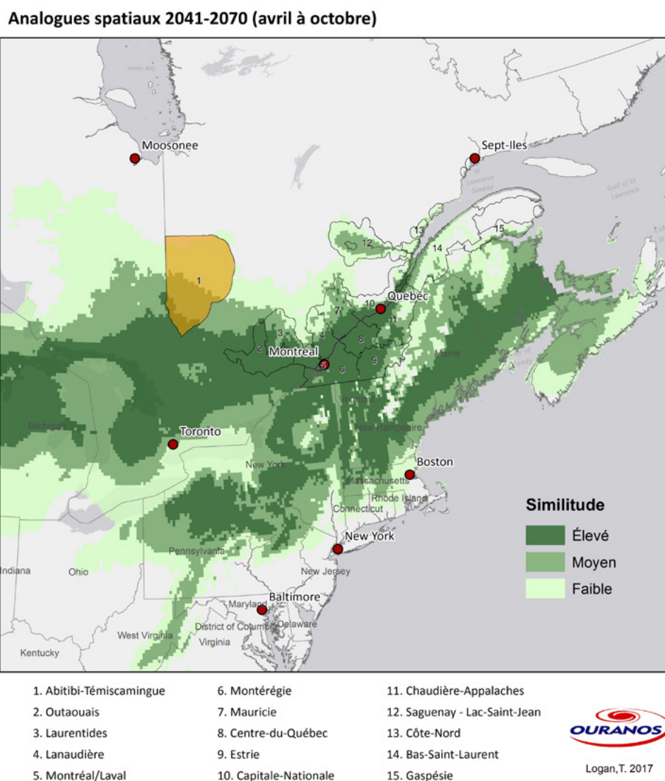
Figure 6 : analogues spatiaux du climat de l'Abitibi-Témiscamingue établi pour la période 2041-2070.
