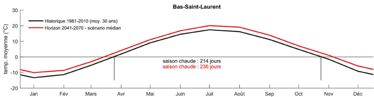
Figure 3 : évolution de la température moyenne mensuelle, en climat historique et futur. La saison dite « chaude », avec une température moyenne supérieure à 0 °C, serait allongée de 22 jours dans le scénario médian.
